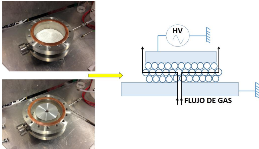
Figura 6. Reactor de placas plano paralelas en configuración de packed-bed utilizado. A la izquierda tenemos imágenes de la cámara abierta sin electrodo activo (arriba) y con electrodo activo (abajo). A la derecha se presenta un esquema de la sección transversal del reactor.
