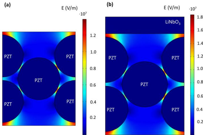
Figura 29. Distribución de campo eléctrico para el reactor estándar (a) y modificado añadiendo una lámina de LiNbO 3 (b). Parámetros de entrada: (a) V = 3 kV, (b) V = 4 kV. Material ferroeléctrico: pellets de PZT.
