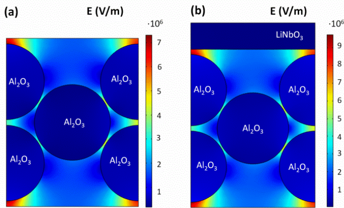
Figura 30. Distribución de campo eléctrico en una barrera packed-bed constituida por pellets de alúmina en el reactor estándar sin (a) y con lámina de ferroeléctrico (b). Tensión aplicada: (a) V = 3 kV, (b) V = 4 kV.
