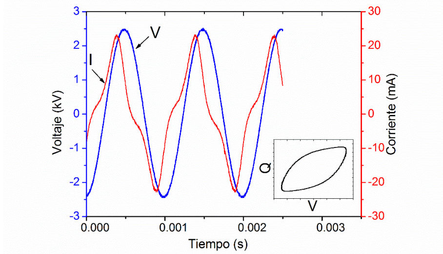
Figura 8. Señales típicas de tensión y de corriente en una descarga DBD en nuestro montaje experimental, y figura de Lissajous correspondiente (abajo a la derecha).
