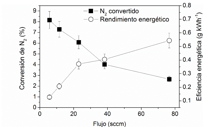
Figura 38. Dependencia de la conversión y de la eficiencia energética con el flujo total de entrada para un voltaje aplicado de 4.1 kV a 5000 Hz, con pellets ferroeléctricos de tamaño 2-3 mm.
