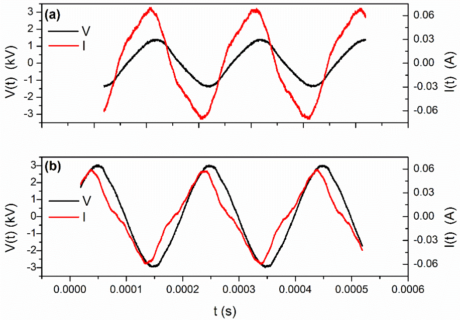
Figura 23. (a) Curvas V(t) e I(t) medidas a 5 kHz en el reactor escalado. (b) Ídem para el reactor estándar. Mezcla gaseosa de entrada: aire seco y metano.
