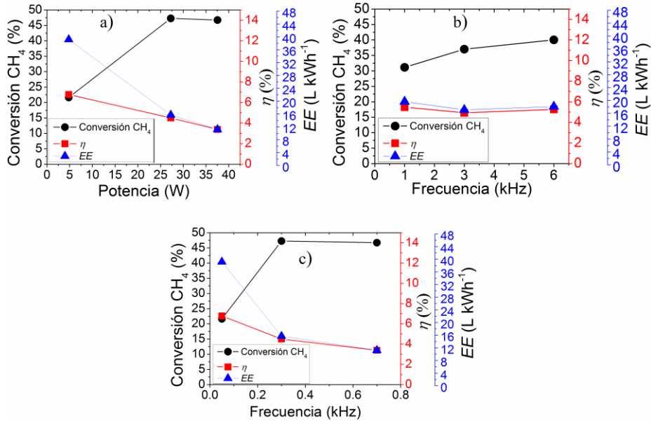
Figura 14. Valores de conversión de metano, EE y eficiencia LHV en función de la potencia y la frecuencia en el reformado oxidativo empleando CH 4 y O 2 como reactivos y pellets de PZT de tamaño 0.5-2 mm como barrera. a) Gráfica en función de la potencia aplicada en una barrera de 10 mm de espesor a frecuencias de 50 Hz (4.8 W), 300 Hz (27.2 W) y 700 Hz (37.5 W). b) Gráfica en función de la frecuencia en una barrera de 3 mm de espesor. c) Ídem para una barrera de 10 mm de espesor.
