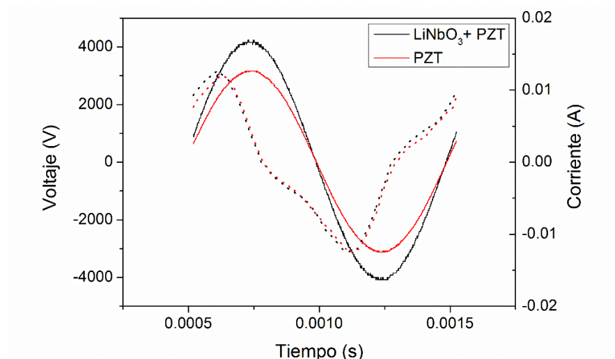
Figura 28. Curvas V(t) e I(t) para el reactor estándar con y sin lámina de niobato de litio. La línea continua corresponde al voltaje y la línea discontinua a la corriente.
