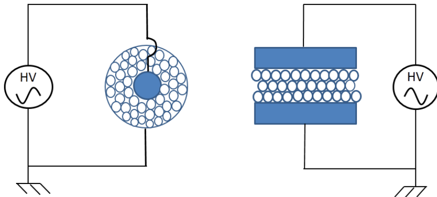
Figura 5. Descarga DBD en configuración de packed-bed con geometrías cilíndrica (izquierda) y plano paralela (derecha).
