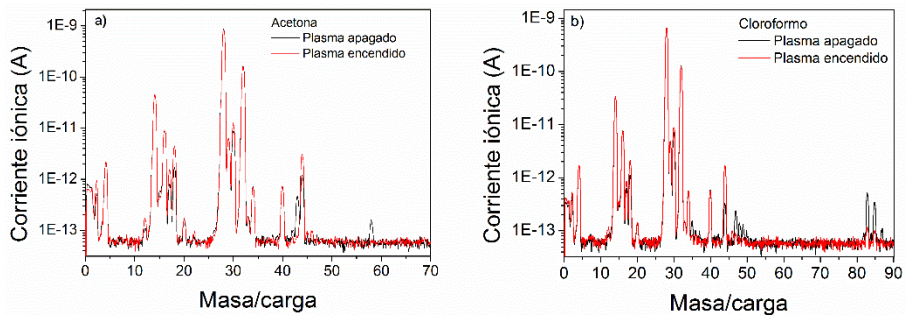
Figura 22. Espectros de masas para un flujo de 300 sccm y a) Acetona o b) Cloroformo como contaminante en el reactor estándar.
