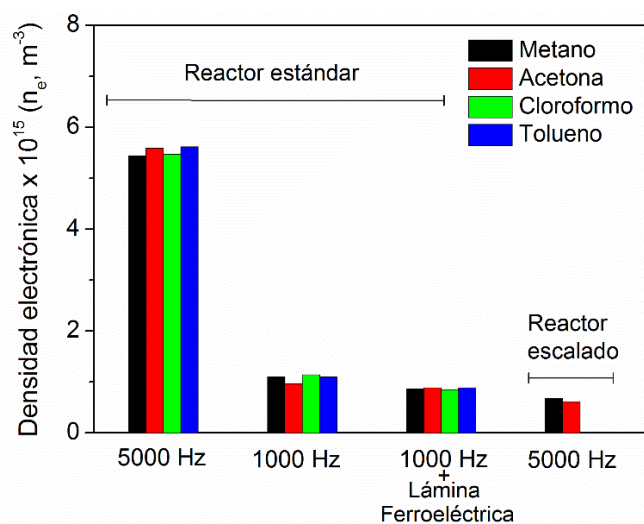
Figura 31. Densidades electrónicas calculadas para diferentes contaminantes y configuraciones de reactor tal y como se indica en la gráfica (flujo total: 100 sccm).
