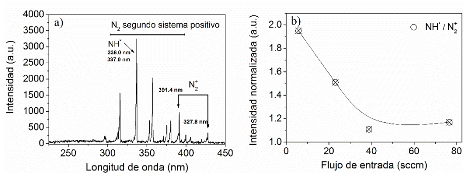
Figura 39. a) Espectros de emisión óptica recogidos a 4.1 kV y 5000 Hz. b) Intensidad normalizada a N_2^+ conforme el tiempo de residencia del gas disminuye. El espesor de barrera es de 10 mm y el tamaño de pellet 2-3 mm.
