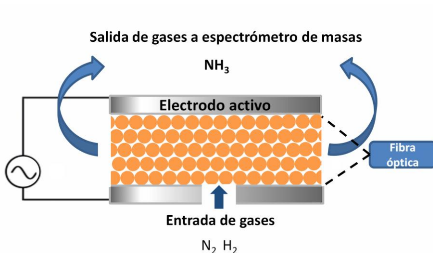
Figura 32. Esquema del montaje experimental empleado en la producción de amoníaco.
