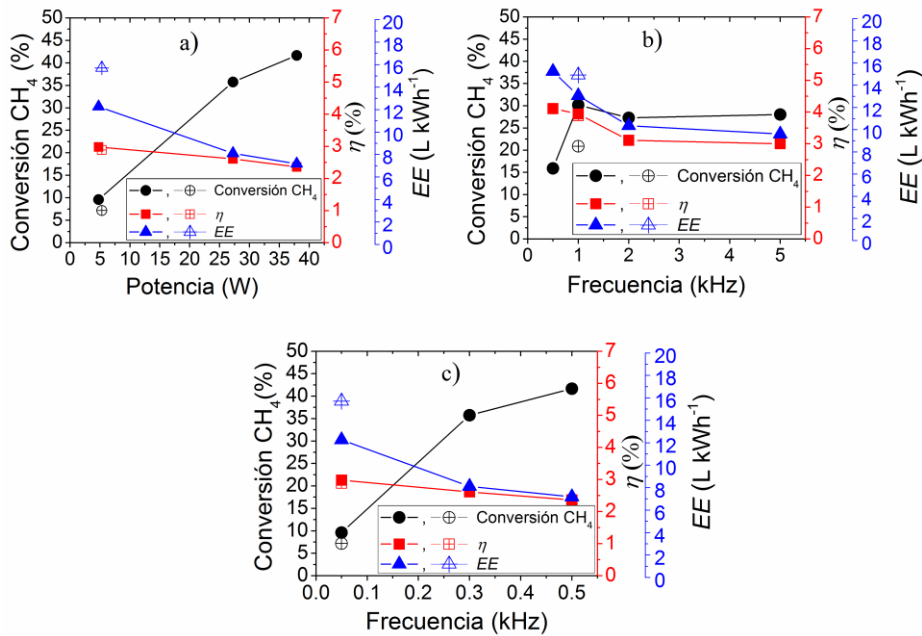
Figura 13. Conversión de metano, EE y eficiencia LHV en función de la potencia y la frecuencia en el reformado húmedo empleando CH 4 y H 2 O como reactivos y pellets de PZT de tamaño 0.5-2 mm como barrera. a) Gráfica en función de la potencia aplicada en una barrera de 10 mm de espesor a frecuencias de 50 Hz (4.8 W), 300 Hz (27.2 W) y 500 Hz (37.9 W). b) Gráfica en función de la frecuencia en una barrera de 3 mm de espesor. c) Ídem para una barrera de 10 mm de espesor. Los puntos con una cruz representan datos de experimentos con flujo doble de CH 4 y H 2 O.
