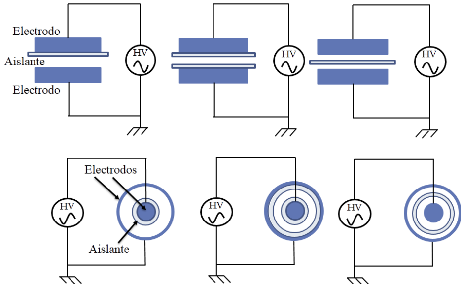
Figura 4. Diferentes configuraciones de una descarga DBD. Se presentan una serie de geometrías plano paralelas (fila superior) y cilíndricas (fila inferior).
