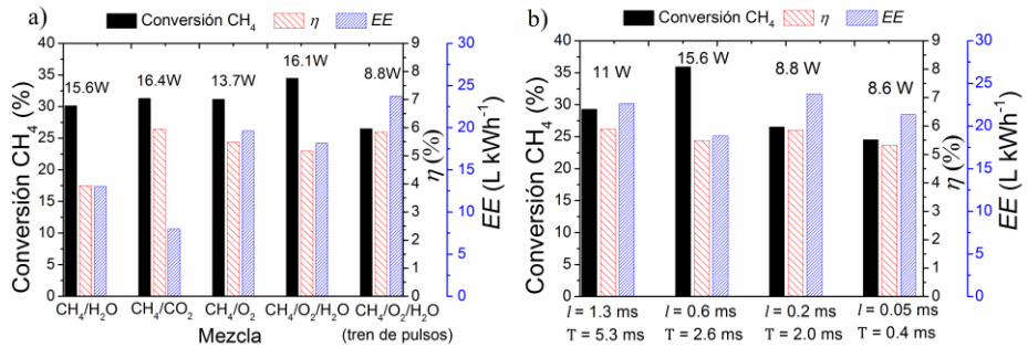
Figura 16. a) Comparación de los mejores resultados obtenidos con diferentes mezclas de reactivos utilizando una barrera de 3 mm de espesor de pellets de PZT con tamaños entre 0.5 y 2 mm. En todos los casos se aplica un voltaje alterno a la frecuencia de 1 kHz excepto en uno, en el que se utiliza un tren de pulsos caracterizado por una longitud de pulso l = 0.2 ms y un periodo T = 2 ms. b) Comparación de resultados conseguidos con la mezcla ternaria y diferentes trenes de pulsos. Todos los datos presentados se obtienen con una barrera de 3 mm de PZT de pellets de tamaños comprendidos entre 0.5 y 2 mm. La potencia aplicada en cada caso se indica en las gráficas.
