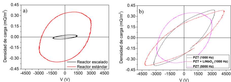
Figura 27. Curvas de Lissajous expresadas en términos de densidad de carga (carga por unidad de área del electrodo) para los reactores y condiciones de trabajo examinados. a) Reactores escalado y estándar trabajando a 5 kHz. b) Reactor estándar con y sin lámina de ferroeléctrico operando a las frecuencias indicadas. Mezcla de gas: aire seco y metano.
