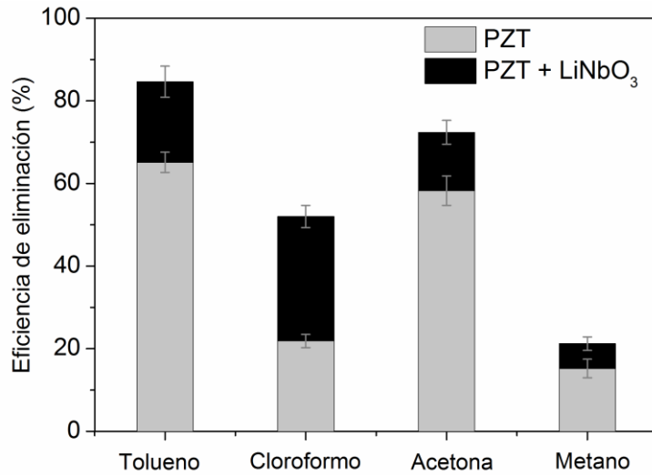
Figura 26. Comparación de los porcentajes de eliminación de los contaminantes estudiados descompuestos en el reactor estándar a 1 kHz con y sin lámina de ferroeléctrico LiNbO 3 (flujo: 100 sccm, tiempo de residencia: 2 s).
