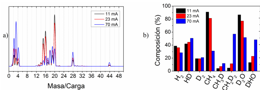
Figura 18. a) Conjunto de espectros de masas recogidos en la reacción de reformado húmedo a corrientes crecientes utilizando \text{D}_2\text{O} y \text{CH}_4 como reactivos. b) Porcentaje de las distintas moléculas marcadas detectadas en el gas de salida en función de la corriente aplicada.
