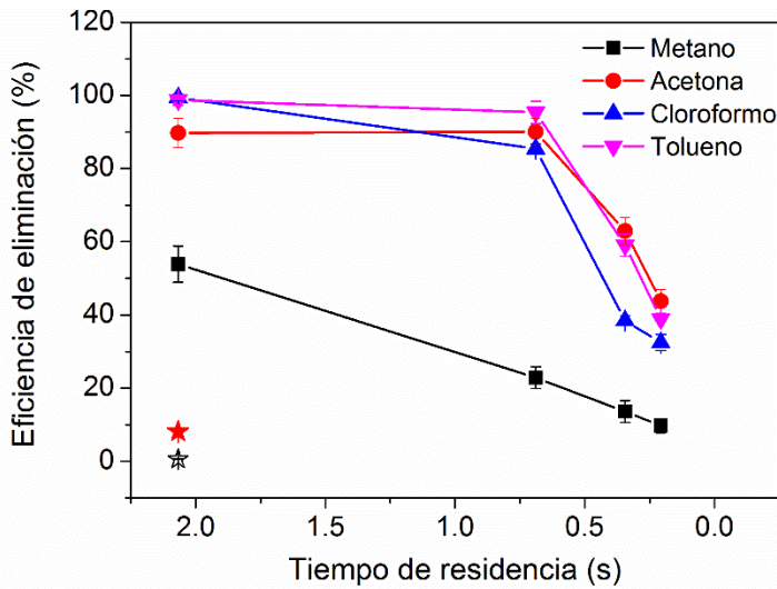
Figura 25. Representación de los porcentajes de eliminación de VOC/metano en función del tiempo de residencia para los cuatro contaminantes elegidos para el análisis. Se presentan datos procedentes del reactor estándar (puntos unidos con líneas) y del reactor escalado (estrellas) a 5 kHz. Las estrellas rellenas y huecas corresponden a acetona y metano, respectivamente.
