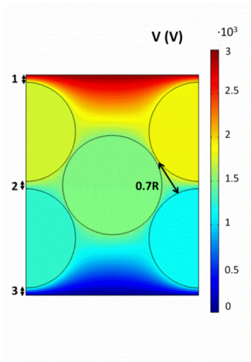
Figura 24. Caída de tensión en una barrera ferroeléctrica constituida por dos capas de pellets ferroeléctricos. Se indican explícitamente las tres regiones de plasma en las que se produce la caída de tensión, señaladas como “1”, “2” y “3”. La máxima separación entre pellets es de 0.7R , siendo R el radio de los mismos. El voltaje externo aplicado es de 3 kV.
