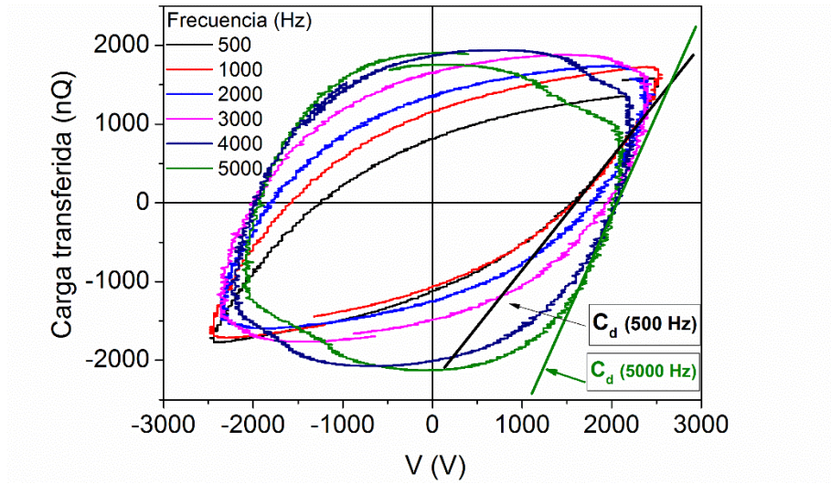
Figura 35. Curvas de Lissajous para el reactor trabajando a las frecuencias indicadas con una barrera de 3 mm de espesor, pellets de tamaño 0.5-2 mm y un voltaje de 2.5 kV. Las líneas rectas dibujadas en la figura se usan para determinar la capacidad del sistema según la referencia [80].
