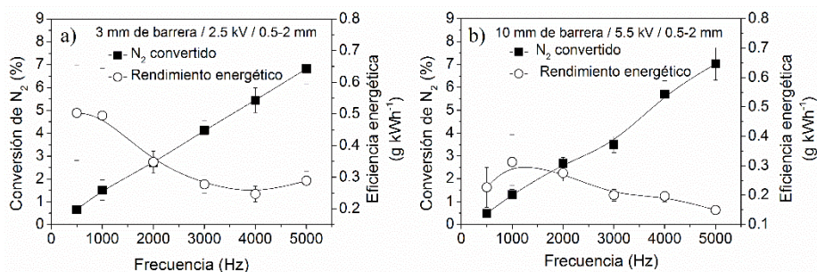
Figura 33. Conversión de N_2 y eficiencia energética en función de la frecuencia. Los espesores de barrera son 3 mm en a) y 10 mm en b), con tensiones aplicadas de 2.5 kV y 5.5 kV, respectivamente. El tamaño de los pellets se encuentra en un rango 0.5-2 mm.
