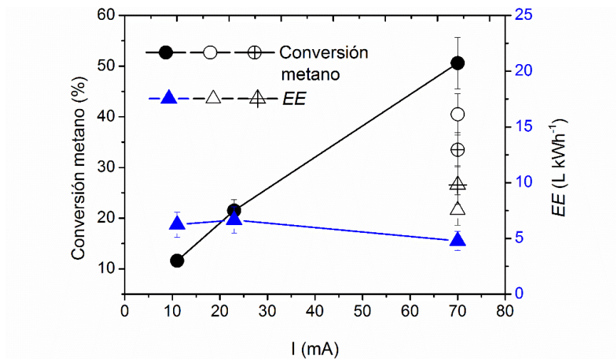
Figura 17. Conversión de metano y eficiencia energética en el reformado húmedo de metano con D 2 O en función de la corriente aplicada, con un flujo total de entrada de 13.8 cm 3 min -1 (símbolos rellenos). Los datos correspondientes a experimentos doblando el flujo total de los reactivos se representan con símbolos huecos y los obtenidos triplicando el flujo total con símbolos con cruz.
